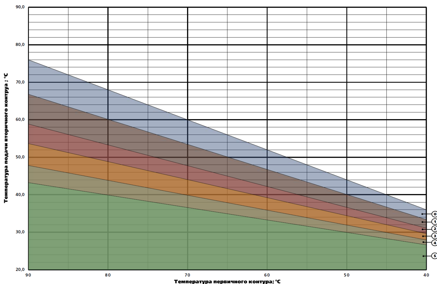
График настройки смесительного клапана
